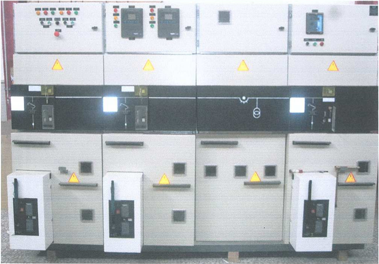
تابلو فشار متوسط چنج اوور با کنترلر اتوماتیک Sepam.B21 اشنایدر
